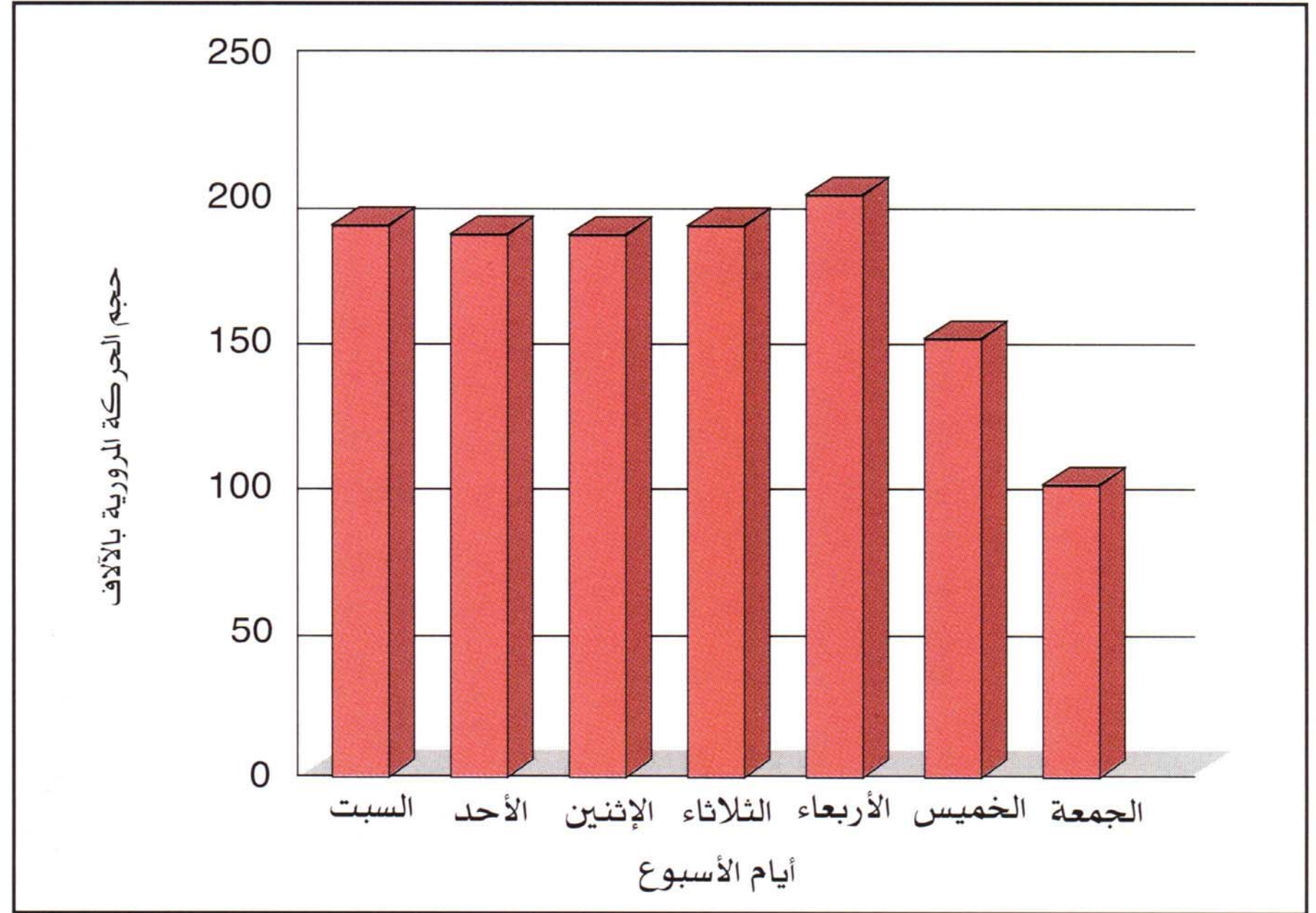
متوسط حجم الحركة المرورية اليومية لمختلف أيام الأسبوع في مدينة الرياض
